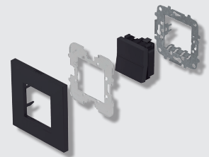
Explosionado Marco IP44
