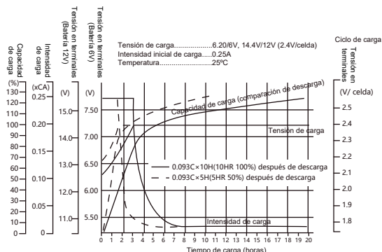
Curva de GL en tensión constante
