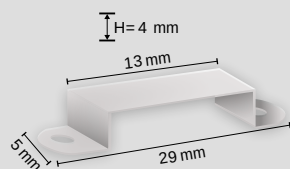
2490032 Clip de sujeción Clípe de fixação | Mounting clip
