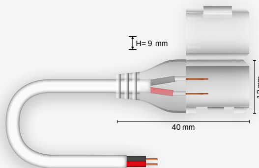
2490035 Cable conexión Cabo de ligação | Connection Cable
