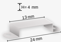
2490031 Clip de sujeción Clípe de fixação | Mounting clip
