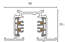
CARRIL TRIFÁSICO EMPOTRAR DE 2 METROS NEGRO CÓDIGO: 62500 BLANCO CÓDIGO: 62502 PVP: 101,50€
