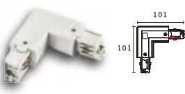
CONECTOR EN "L" DERECHA NEGRO CÓDIGO: 62536 BLANCO CÓDIGO: 62537 PVP: 32,95€
