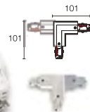
CONECTOR EN "L" REVERSIBLE (IZQ.-DER.) NEGRO CÓDIGO: 62528 BLANCO CÓDIGO: 62529 PVP: 36,50€
