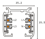
CARRIL TRIFÁSICO SUPERFICIE DE 2 METROS NEGRO CÓDIGO: 62504 BLANCO CÓDIGO: 62506 PVP: 76,50€
