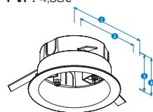
1. 130mm 2. 105mm 3. 58mm 4. 60mm ADAPTADOR EMPOTRAR UNITARIO NEGRO CÓDIGO: 62440 BLANCO CÓDIGO: 62441 PVP: 40,90€
